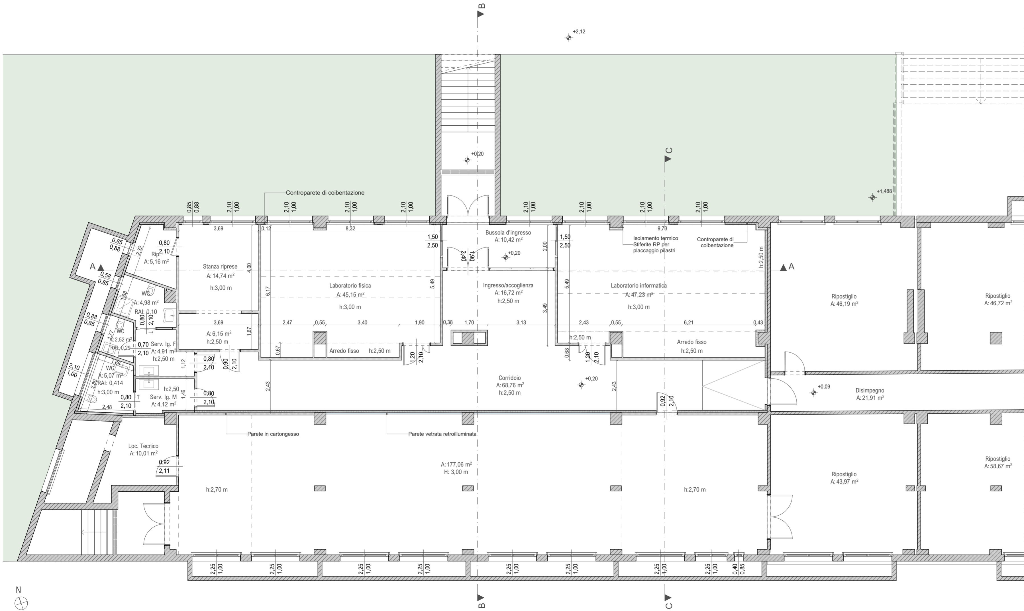
PIANTA DI PROGETTO
